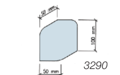
Esquinero vertical para zócalo de 100 x 200 mm
