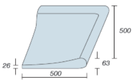
3 Esquina invertida r = 0
