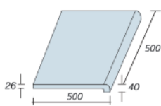
8 Loseta con terminación
